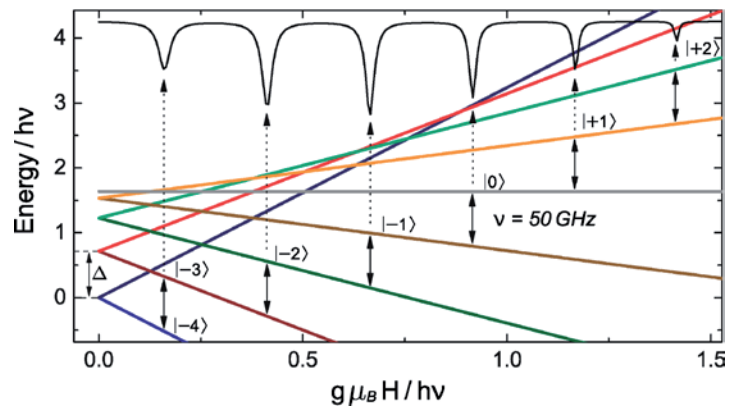
Abb.: Zentrales Gerüst eines vierkernigen Ni(II)-Komplexes mit einem bistabilem High-Spin-Grundzustand von S=4 und einer negativen magnetischen Anisotropie ( D_{\text{mol}}=-0.31 K). Rechts: Spin-Zustände des Komplexes in einem externen Feld H (parallel zur magnetischen Anisotropie Achse) sowie simuliertes HF-ESR-Spektrum.
