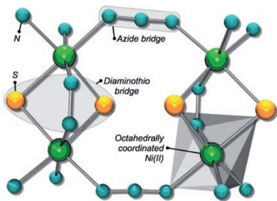
Abb.: Zentrales Gerüst eines vierkernigen Ni(II)-Komplexes mit einem bistabilem High-Spin-Grundzustand von S=4 und einer negativen magnetischen Anisotropie ( D_{\text{mol}}=-0.31 K). Rechts: Spin-Zustände des Komplexes in einem externen Feld H (parallel zur magnetischen Anisotropie Achse) sowie simuliertes HF-ESR-Spektrum.
