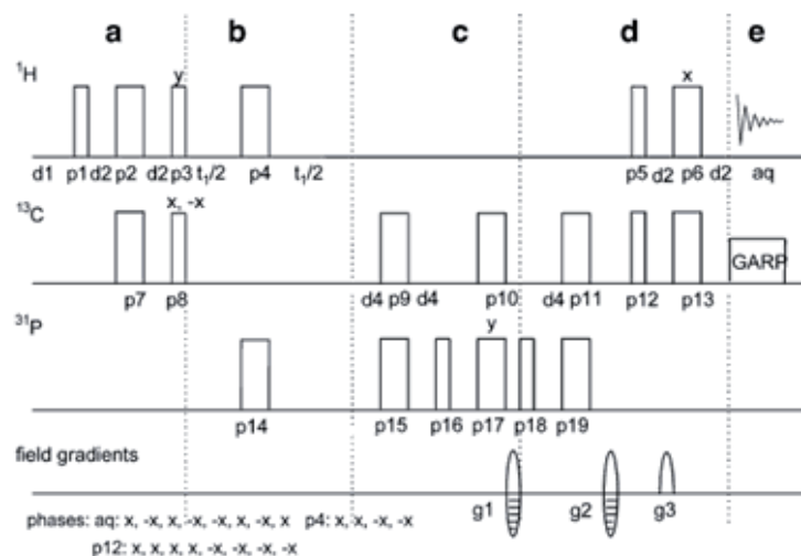
Abb.: NMR-Pulssequenz zur Kontrolle der Phosphorylierung von Peptiden
